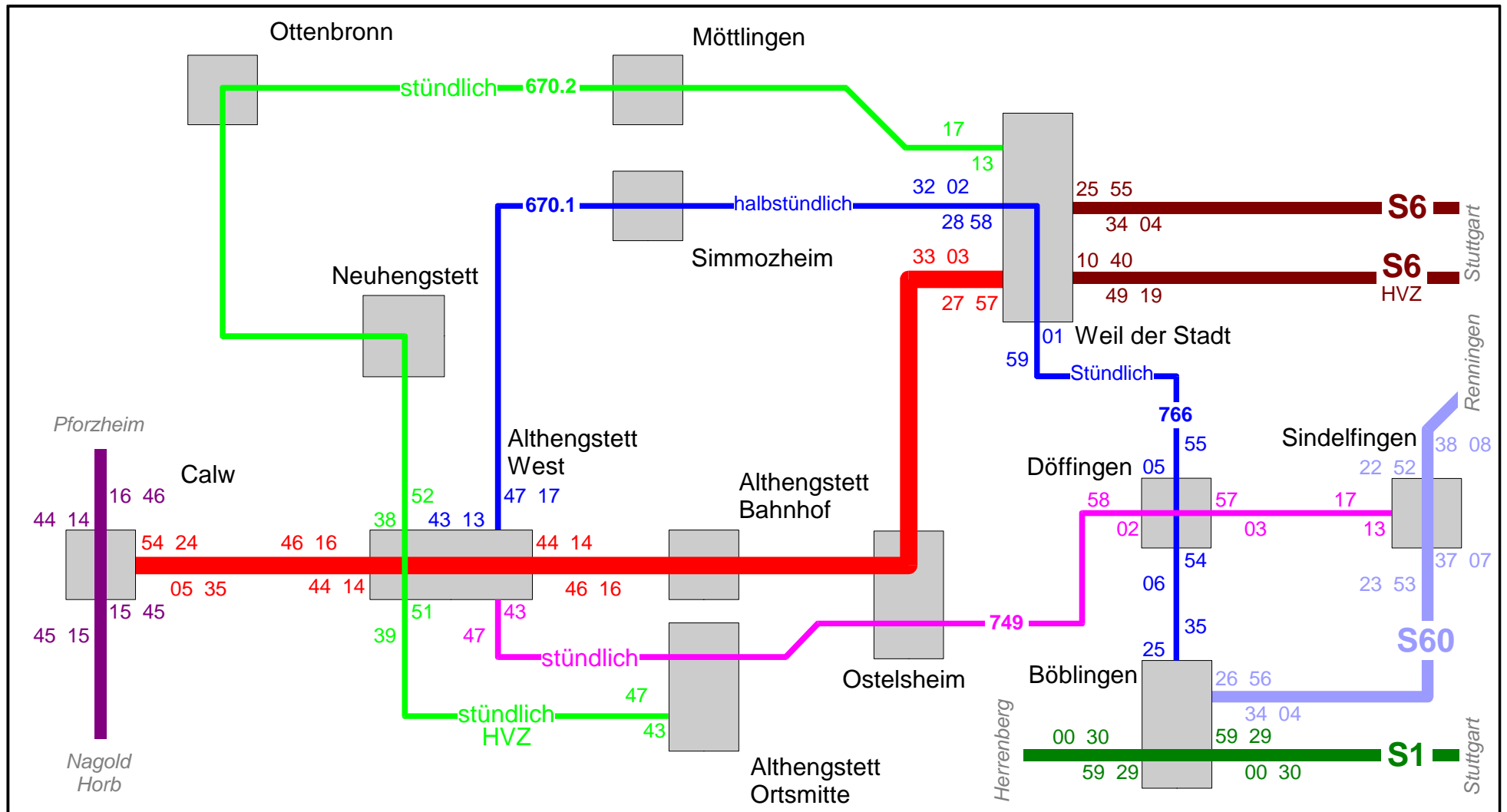
Schienenverbindung Calw - Weil der Stadt Angebotskonzept im Korridor Calw - Weil der Stadt Netzgrafik für die Hauptverkehrszeit HVZ
